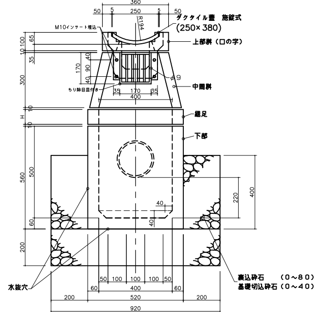
A-A断面図
