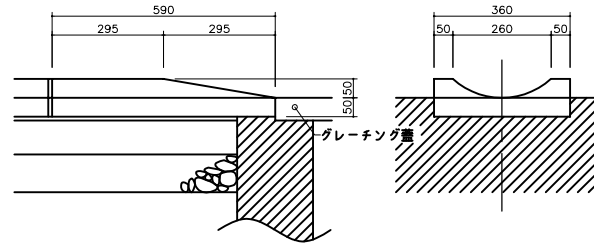
A-A断面図
