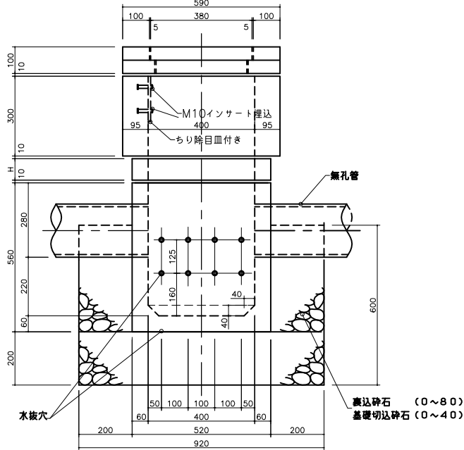
側面図
