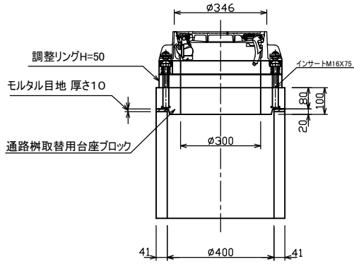
台座ブロック製品図
