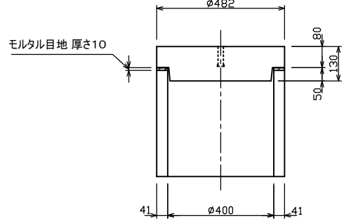
閉塞蓋製品図
