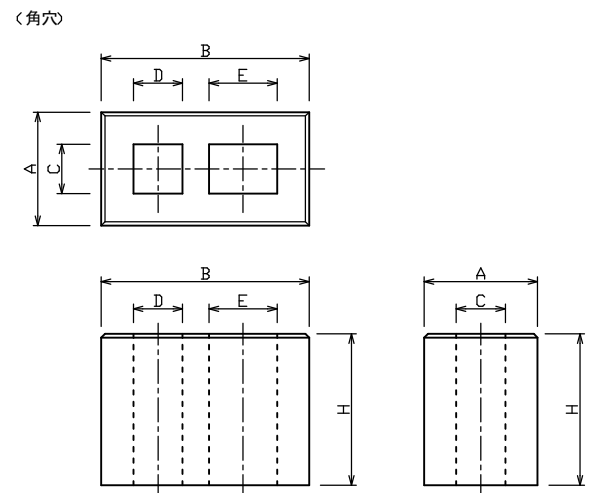
角穴 2つ穴 単位 (mm)
