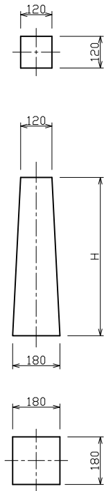
標準型
