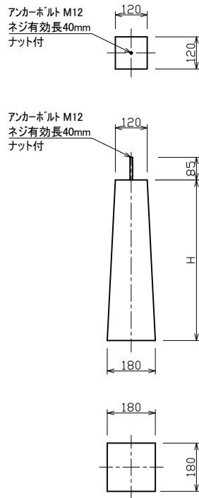
アンカーボルト型
