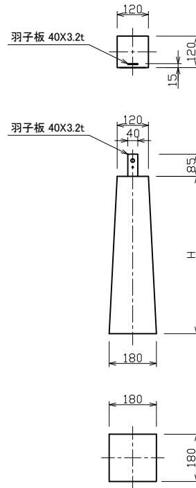
羽子板型
