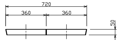
蓋 (1枚当たり) 標準重量 W=31 (kg)
