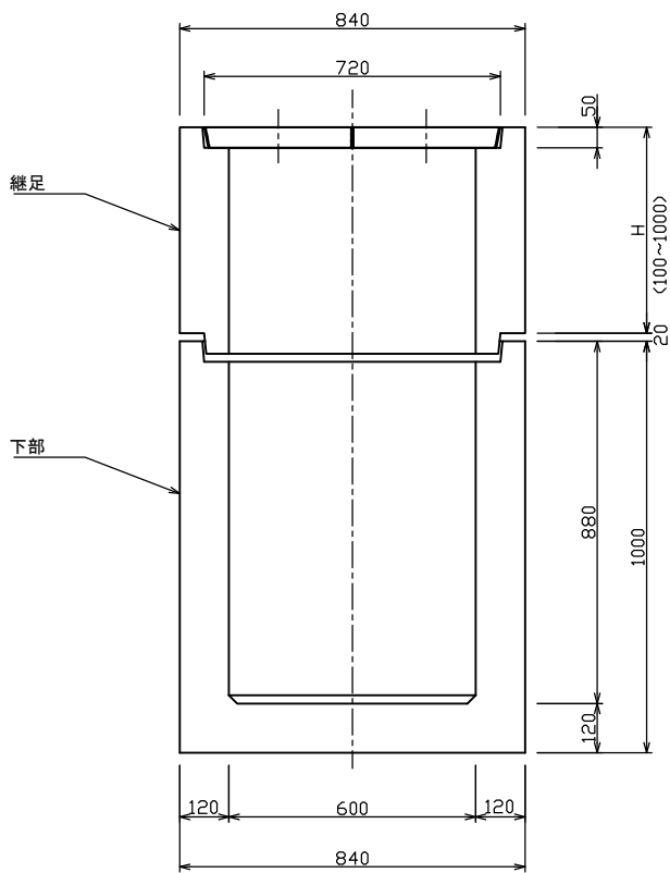
標準重量 W= 83 (kg) (H=100当たり)
