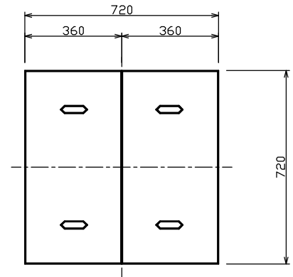
鉄板巻コンクリート蓋
