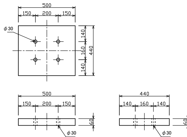
消火栓用台座
