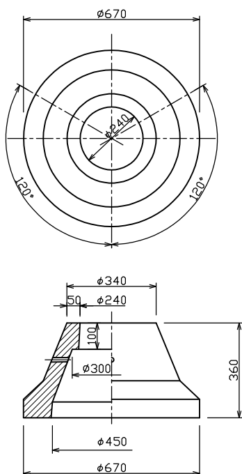
仕切弁筐(朝顔) A型
