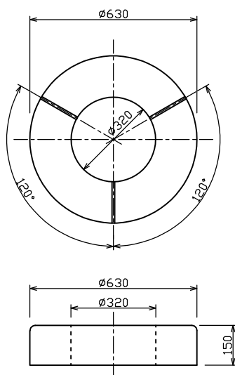
縁石(仕切弁用メガネ石)
