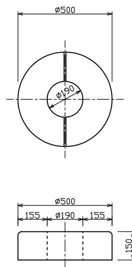
消火栓用メガネ石(2つ割)
