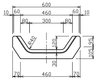
皿型側溝 T-5 H=120(学校用)
