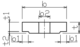
水抜き用切欠き有り
