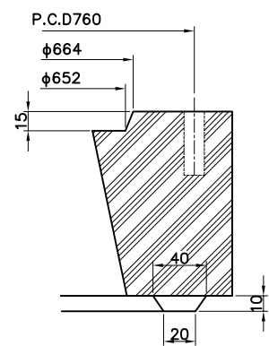
接合目地詳細図
