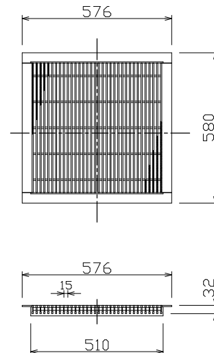
グレーチング(細目)
