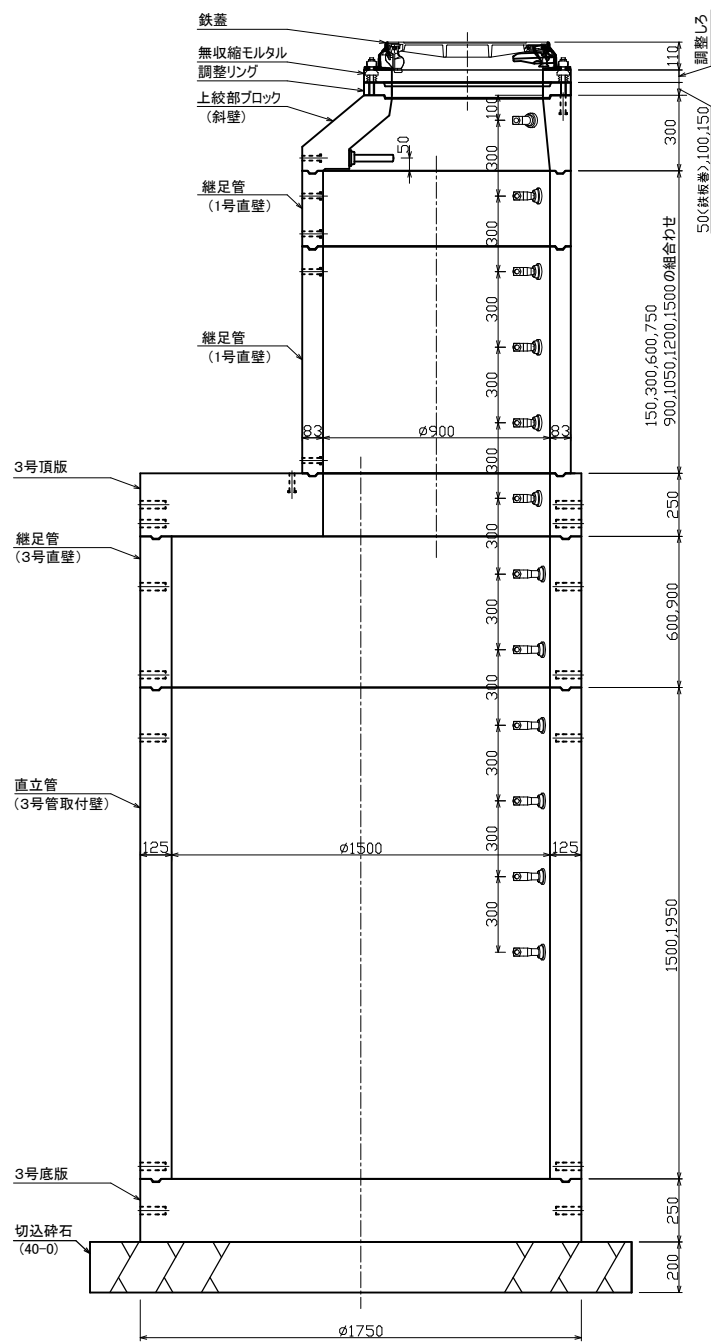
(札幌市型)3号型マンホール標準図
