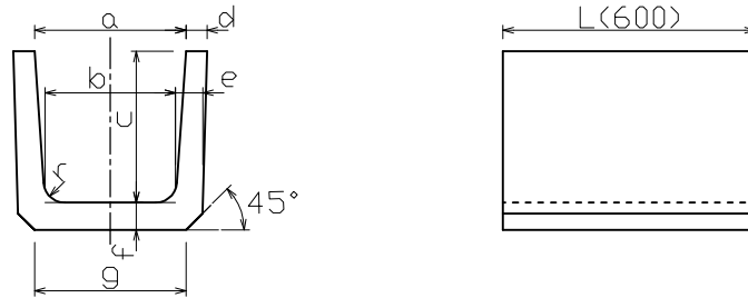
(JIS A 5372 推奨仕様 E-1)
