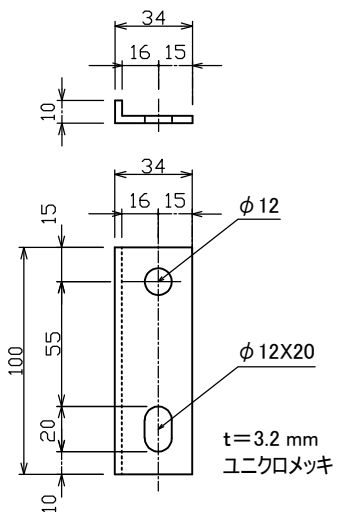
固定金具詳細図 (S=1/5)
