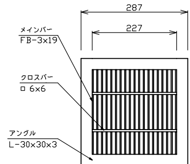
グレーチング (細目)
