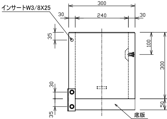
固定金具詳細図 (S=1/5)
