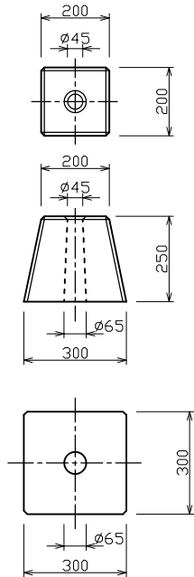
E型(スノーポール基礎)
