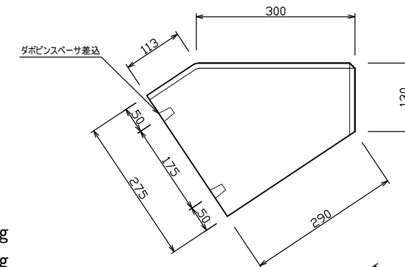
中段ブロック(1段あたり)
