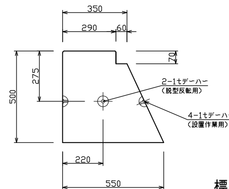
法留めブロック(ノスキッド加工)
