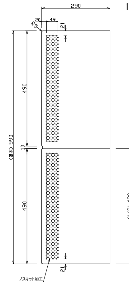
法留めブロック(ノスキッド加工)
