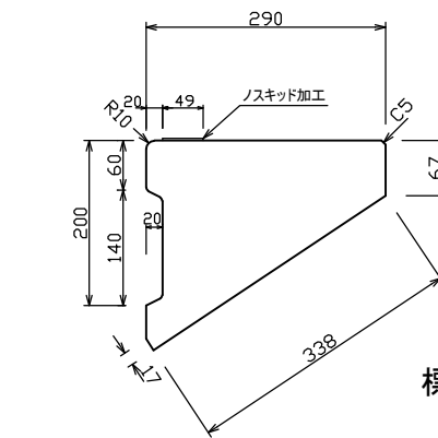
本体ブロック
