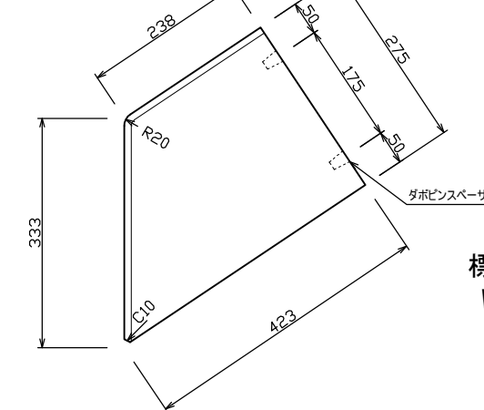
下段ブロック
